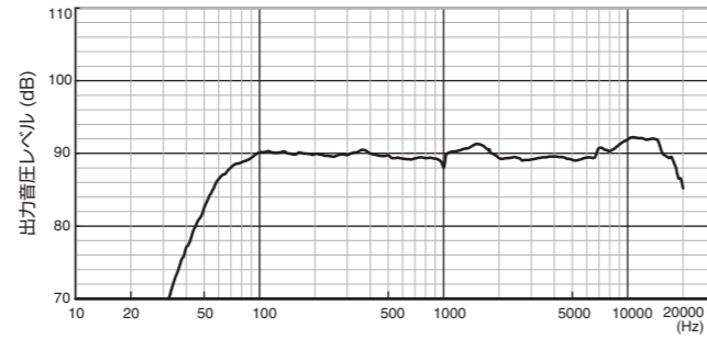
出力音圧周波数特性 (FLAT ポジション)
