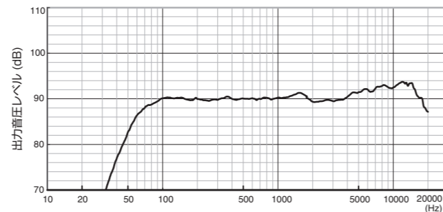
出力音圧周波数特性 (TREBLE ポジション)
