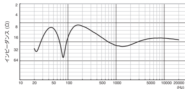
インピーダンス特性
